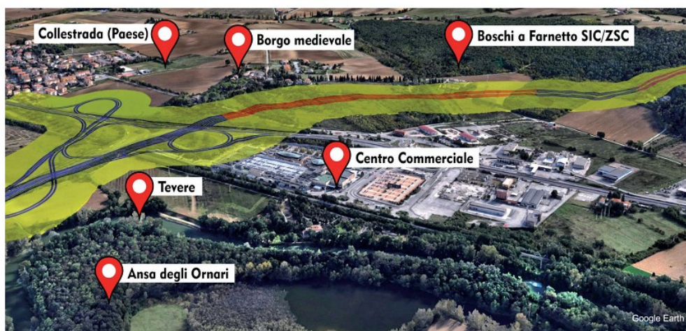
■ sede stradale fuori terra ■ galleria artificiale ■ galleria Libera elaborazione del progetto preliminare del Nodo di Perugia
